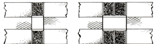
Principedetail brandwerende dilatatievoegen
